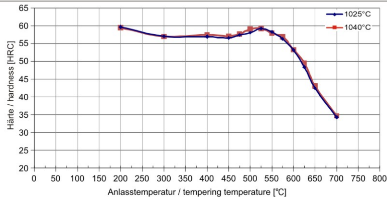
回火曲线图： 试样尺寸为20mm×28mm×36mm；淬火温度1025℃和1040℃（1个小时），风冷
